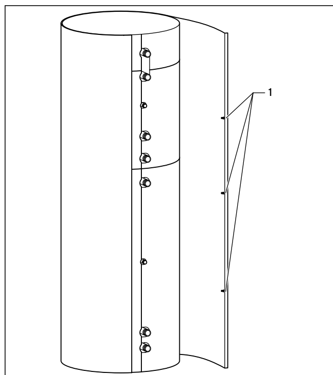
Fig. 5.9 Dévisser l'habillage
